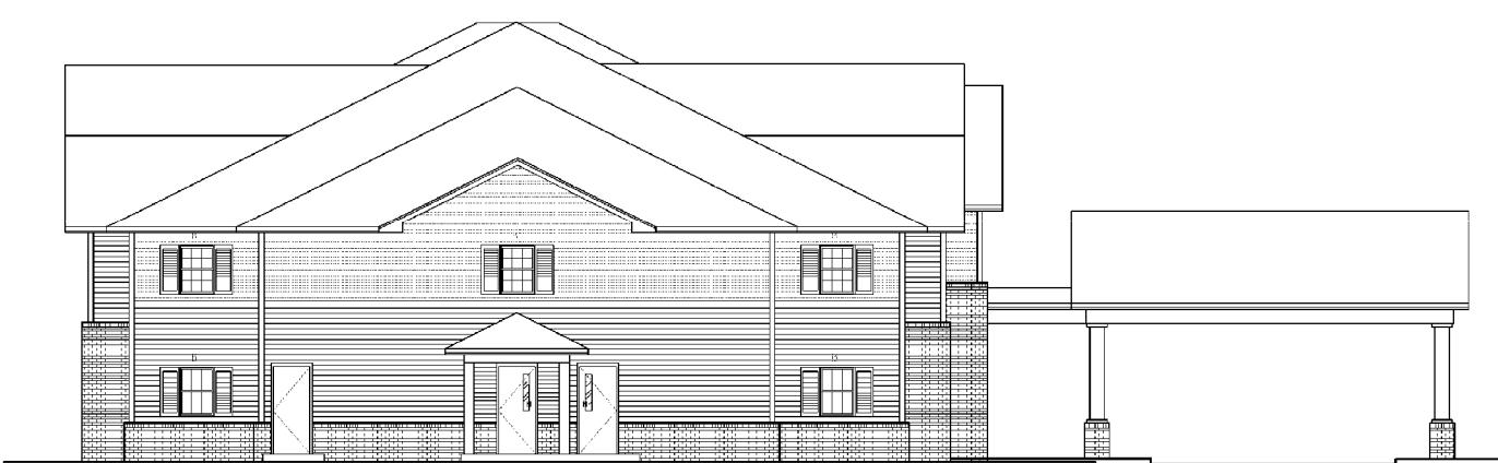
03 SIDE ELEVATION A5.02 SCALE: 1/8" = 1'-0"
